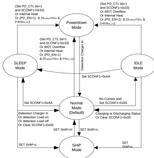
图5 模式转换图
