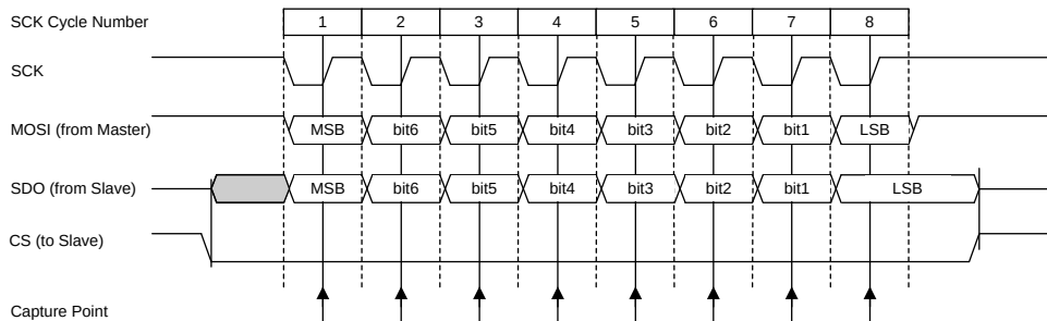
数据传送形式 (CPHA = 1, CPOL=1)
