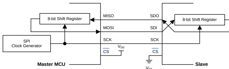
全双工主从互联图
